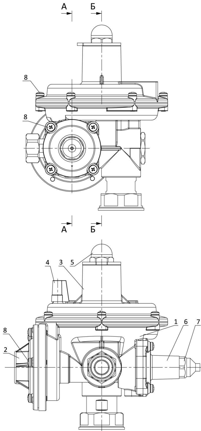
Рисунок 1 – Устройство регулятора давления «РЕД-2»
